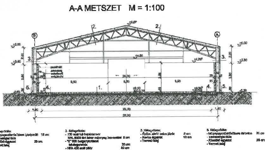
Építész metszet, forrás: építész tervező
