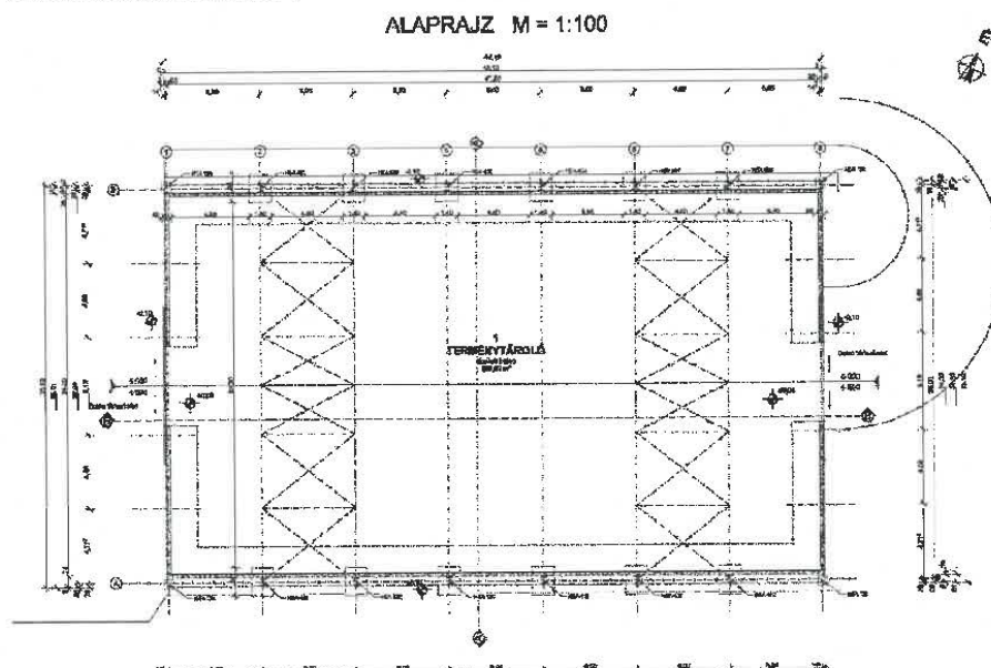
Építész alaprajz, forrás: építész tervező
